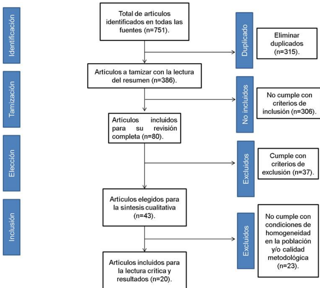
Figura 1. Esquema PRISMA.
