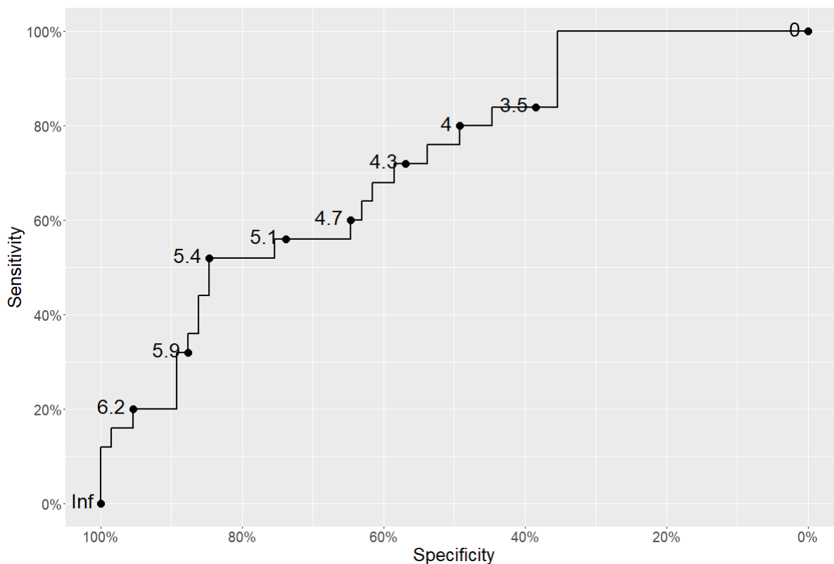
Figura S1. Curva ROC (Receiver Operating Characteristic). La curva ROC fue generada a partir de la cuantificación de Campylobacter (GC/g) en muestras de pollo de mercados tradicionales utilizando qPCR. Al maximizar la suma de sensibilidad y especificidad, se estableció un punto de corte óptimo de 5.37 log 10 GC/g, en función de los resultados de cultivo.
