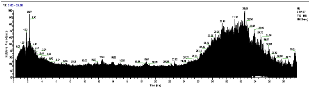
Figura 7.- Cromatogramas en el modo negativo del Residuo butanólico (RBUT)
