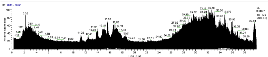
Figura 8. Cromatogramas en el modo negativo de la fracción obtenida con 50% de acetonitrilo del residuo butanólico del extracto etanólico (50% ACN del RBUT del EtOH) de la tara
