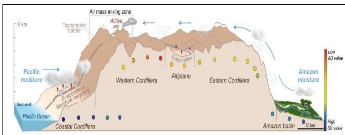
Figura 44. Esquema de los Andes Centrales del Perú que muestra los procesos climáticos que influyen en la distribución espacial moderna de los valores isotópicos. Fuente: White et al., 2024.
