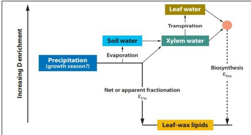
Figura 10. Diagrama conceptual que describe las relaciones isotópicas de hidrógeno entre la precipitación y los n-alcenos de cera en hojas de plantas terrestres (no a escala). El punto rojo ilustra una reserva de agua biosintética hipotética, es decir, una mezcla potencial de diferentes reservas de agua dentro de la hoja y la última fuente de hidrógeno para la biosíntesis de lípidos. Modificado de Sachse et al. (2006) y Smith & Freeman (2006). Abreviaturas: \epsilon_{\text{bio}} , fraccionamiento isotópico de hidrógeno biosintético; \epsilon_{l/w} , fraccionamiento isotópico entre lípidos y agua de origen. Fuente: (Sachse et al., 2012)
