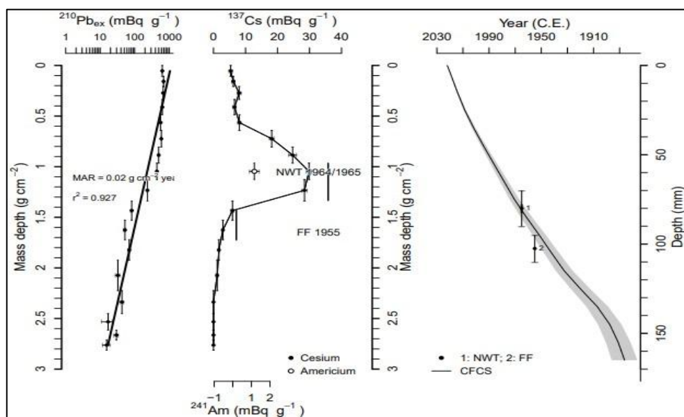
Figura 30. Modelo de Edad de los 17cm superiores en el testigo CHA21-4, basado en la actividad radioactiva de ^{210}\text{Pb} y ^{137}\text{Cs} . Producido por A. Foucher (LSCE, Francia).
