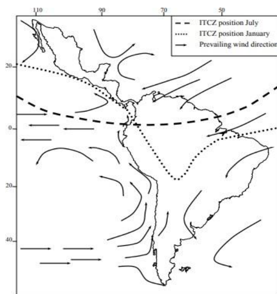
Figura 56. Mapa de Latino América mostrando la presente – posición diaria en verano e invierno de la ZCIT y el patrón de los vientos en macroescala (de ahí la humedad) sobre Latinoamérica. Modificado de Marchant et al., (2009).
