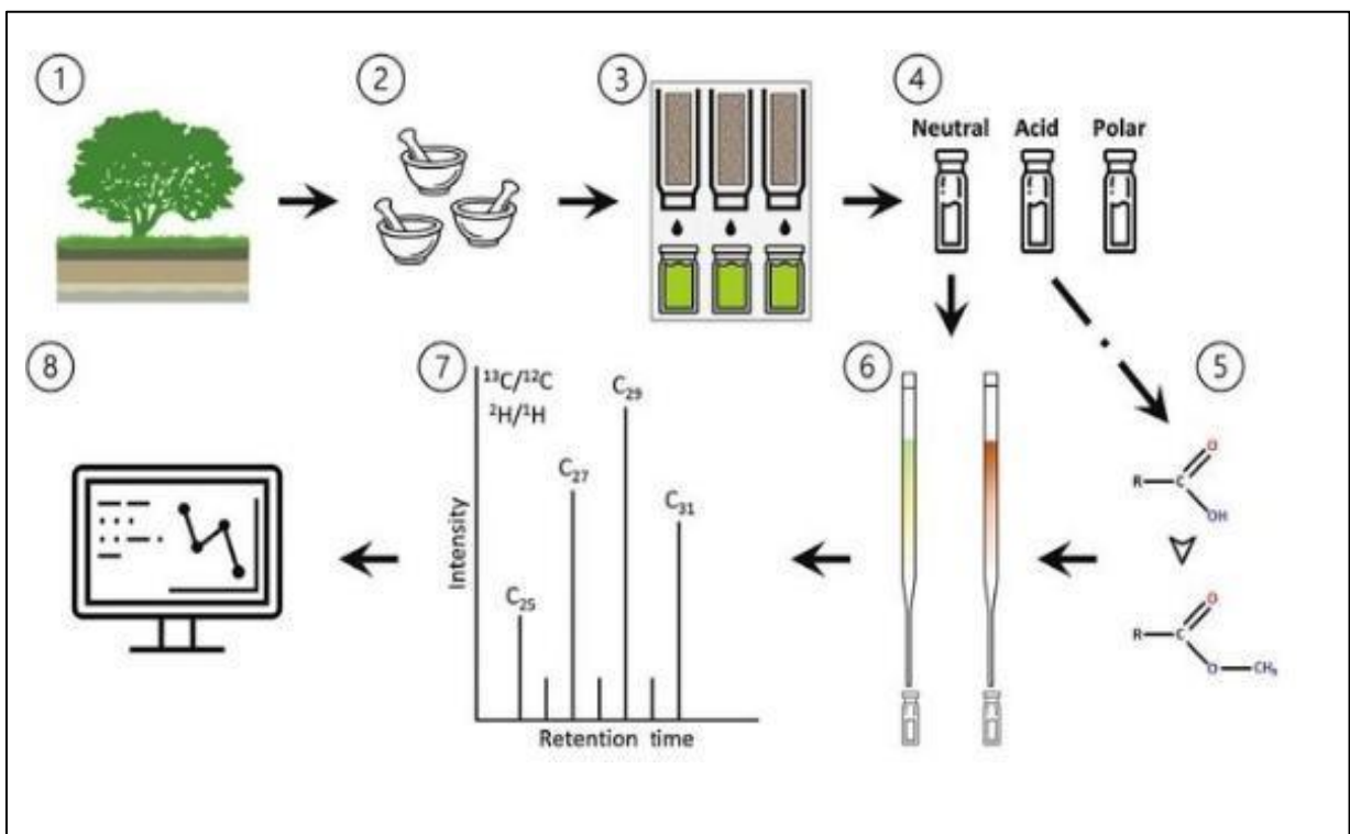
Figura 18. Flujo de trabajo de extracción y análisis de lípidos de cera de hoja para aplicaciones paleológicas. (Patalano et al., 2021)
