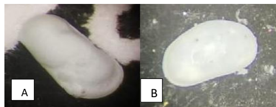
Figura 51. (A) Cytherideidae (género Cyprideis ) y (B) Leptocytheridae (género Leptocythere ).
