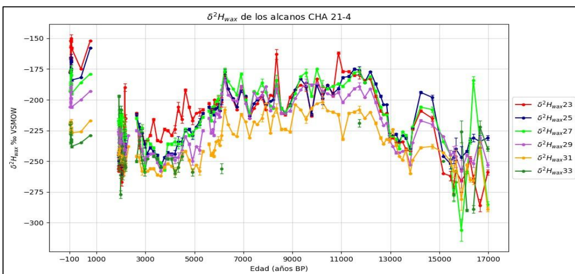
Figura 38. Serie de tiempo de la composición del isotopo estable ^2H del registro CHA - 21-4 en los últimos 17000 años. Donde: \delta^2H_{wax23} (rojo), \delta^2H_{wax25} (azul), \delta^2H_{wax27} (verde claro), \delta^2H_{wax29} (violeta), \delta^2H_{wax31} (amarillo), \delta^2H_{wax33} (verde oscuro).
