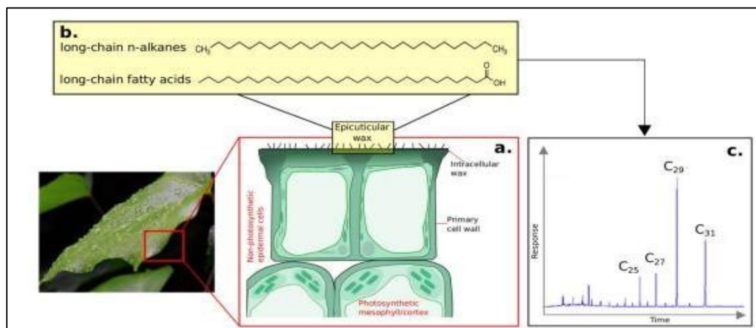
Figura 9. Esquema que muestra la morfología y la química de las ceras epicuticulares de hojas: (a) vista transversal de las células epidérmicas que muestra la cera intracelular y epicuticular, junto con la pared celular y otros arreglos de células fotosintéticas y no fotosintéticas, (b) n-alcenos de cadena larga y ácidos grasos, compuestos ubicuos en las ceras de las hojas de las plantas superiores terrestres; y (c) cromatograma típico de n-alcenos cera de hoja de plantas superiores terrestres que muestra la distribución de homólogos de cadena larga. Fuente: Eley & Hren, (2018)
