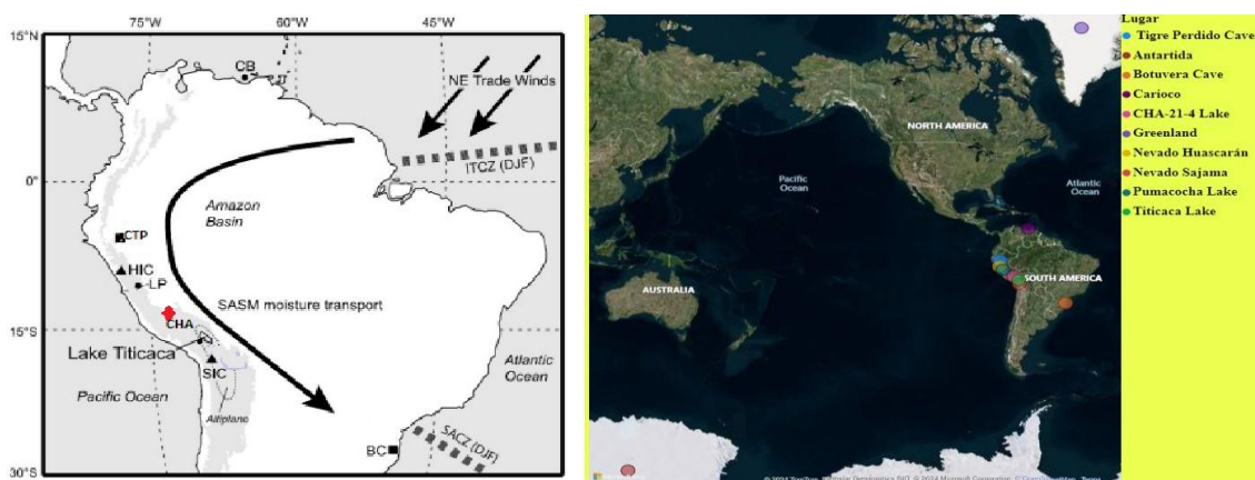
Figura 52. Mapa de Suramérica con la ubicación del registro CHA y otros registros en discusión: espeleotemas (cuadrados), Núcleos de Hielo (triángulos), sedimentos lacustres (círculos) y sitio de estudio (diamante). CB: Cuenca Carioco, CTP: Cueva del
