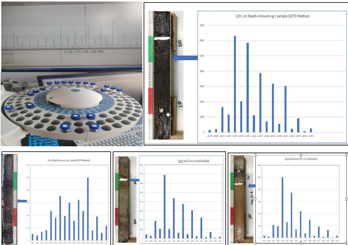
Figura 27. Evaluación de resultados de la CG, concentración y distribución de los n-alcenos.
