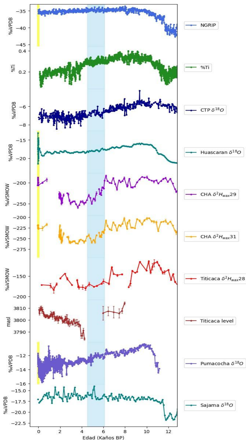
Figura 54. Comparación del registro CHA 21-4 de \delta^2H_{wax29} , \delta^2H_{wax31} con Registro de Groenlandia (NGRIP) ice core \delta^{18}O (Svensson et al., 2008), Registro marino Cuenca del Carioco (%Ti), registro del CTP y Huascarán, del lago Titicaca \delta^2H_{wax28} (Fornace et al., 2014), registro de nivel del lago (Guédron, 2023), registro \delta^{18}O del Pumacocha, y Sajama en los últimos 17 mil años. Franja en azul indica transición, amarilla CM.
