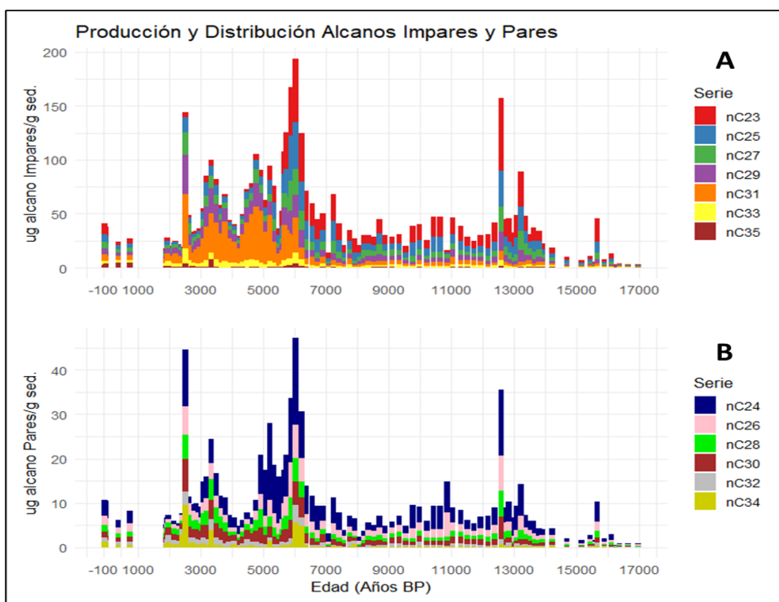
Figura 32. Producción y Distribución de las ceras/lípidos de los alcanos de las plantas, en ug por gramo de sedimento del registro CHA 21-4, a lo largo de los últimos 17 mil años B.P. (A) Serie de alcanos impares (Odd) desde n-C23 al n-C35. (B) Serie de alcanos pares (Even) desde n-C24 al n-C34.
