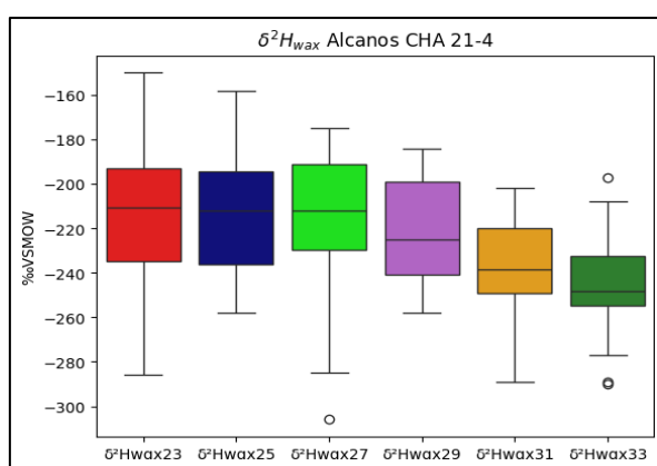
Figura 41. Boxplot del Rango de variación del isotopo estable \delta^2H_{wax} para los alcanos impares del Registro CHA-21-4, a lo largo de los últimos 17000 años B.P.
