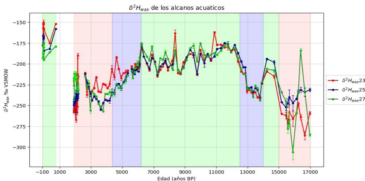
Figura 40. Serie de tiempo del isotopo estable \delta^2H_{wax} de los alcanos terrestres (n-C23, n-C25, n-C27) a lo largo de los últimos 17000 años B.P. del Registro CHA 21-4.
