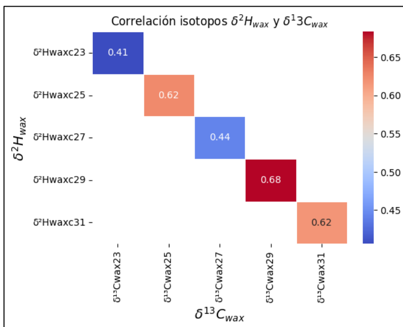
Figura 49. Correlaciones entre \delta^{13}C_{wax} y \delta^2H_{wax} de todos los alcanos en los últimos 17000 años.
