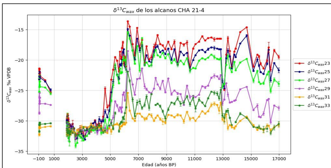
Figura 36. Serie de tiempo de la composición del isótopo estable ^{13}\text{C} del registro CHA - 21-4. de los últimos 17000 años B.P. Donde: \delta^{13}\text{C}_{\text{wax}23} (rojo), \delta^{13}\text{C}_{\text{wax}25} (azul), \delta^{13}\text{C}_{\text{wax}27} (verde claro), \delta^{13}\text{C}_{\text{wax}29} (violeta), \delta^{13}\text{C}_{\text{wax}31} (amarillo), \delta^{13}\text{C}_{\text{wax}33} (verde oscuro).
