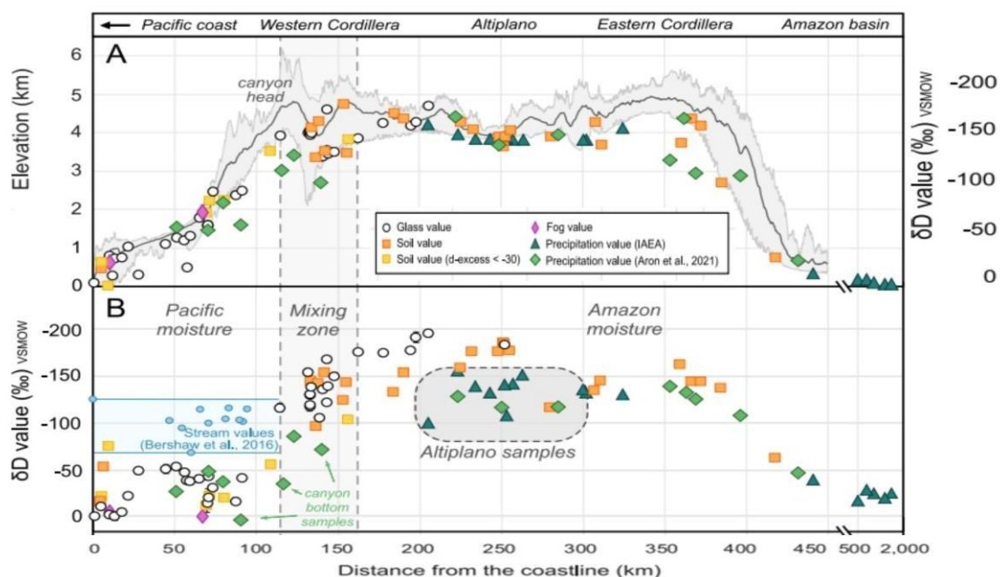
Figura 45. Transectos a lo largo de los Andes Centrales del Perú de (A) Elevaciones de muestra superpuestas en un perfil topográfico moderno y (B) \delta D\text{‰} VSMOW. Modificado de White et al., (2024).
