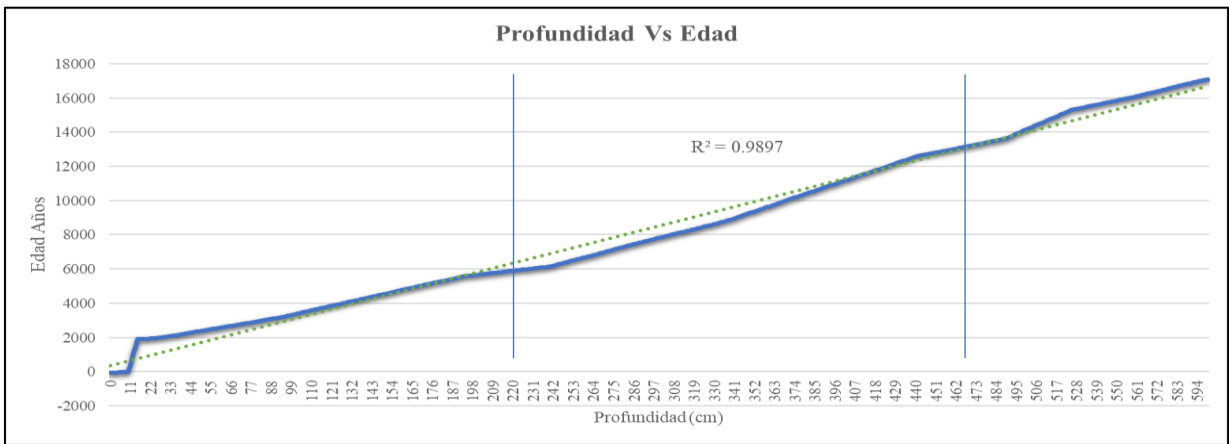
Figura 43. Regresión de data de Profundidad Vs Edad del registro CHA 21-4.
