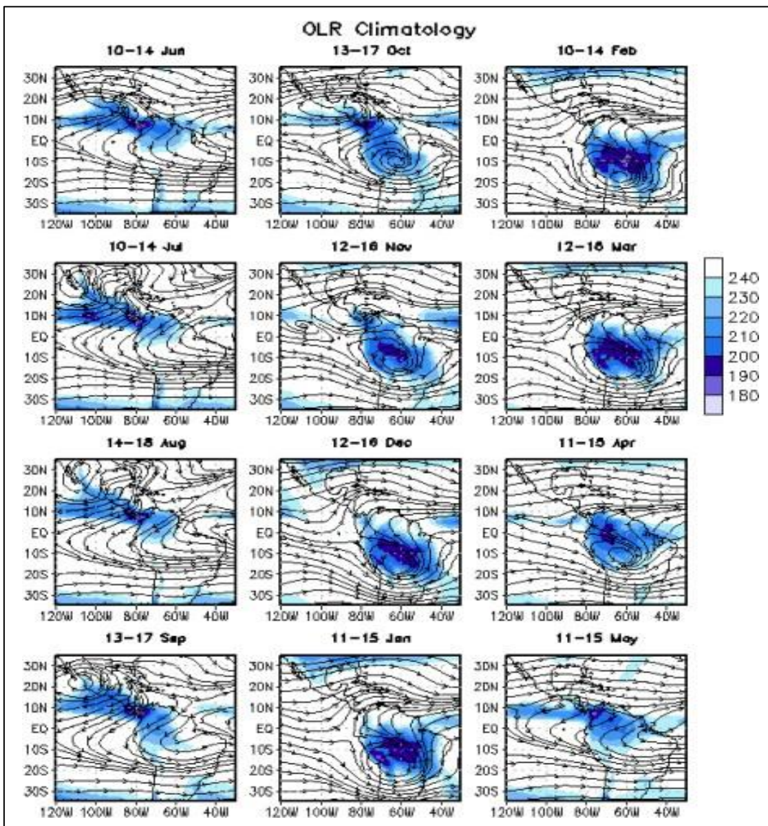
Figura 4. Ciclo estacional promedio de OLR en W/m^2 (1979-1995) y líneas de corriente a 200 hPa. Fuente: Silva y Kousky (2012)
