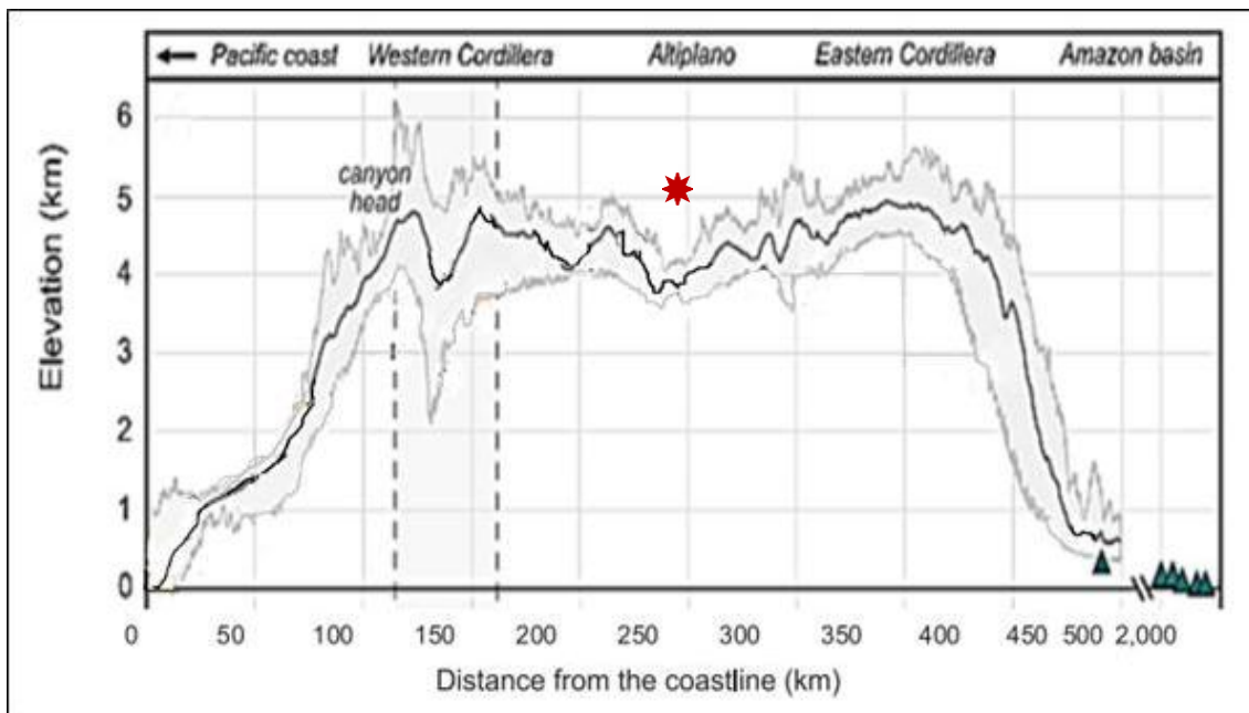
Figura 14. Transectos a lo largo de los Andes Centrales del Perú de elevaciones en un perfil topográfico moderno. Modificado de White et al., (2024). Estrella indica el lugar de estudio.
