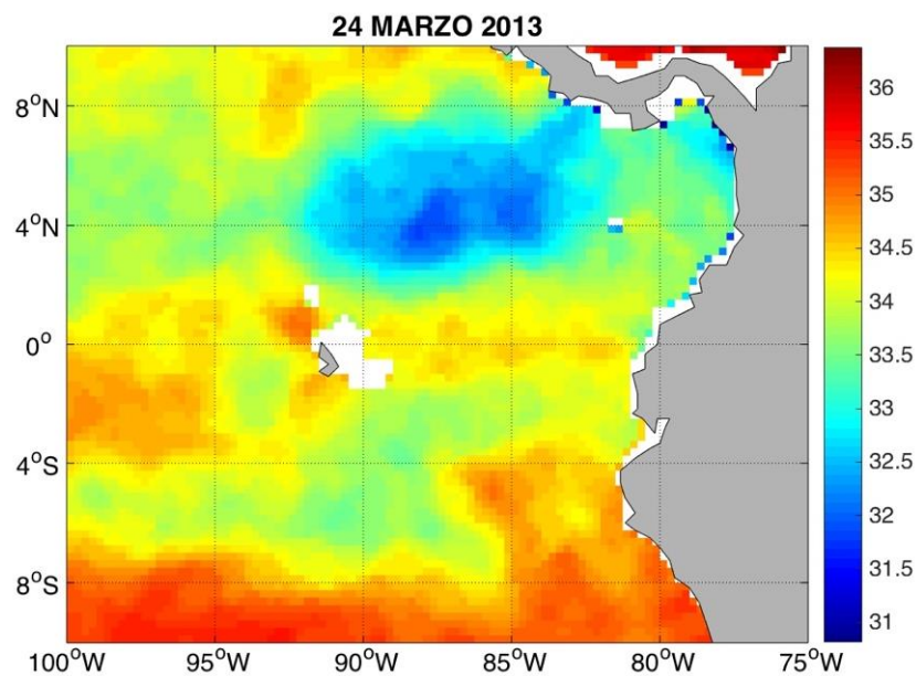
Figura 9. Campo grillado de SSM (en colores) SMOS distribuido por CATDS (producto L3_DEBIAS_LOCEAN_v1) para el día 24 de marzo del 2013 en la región de estudio (100°W-75°W y 10°N-10°S).
