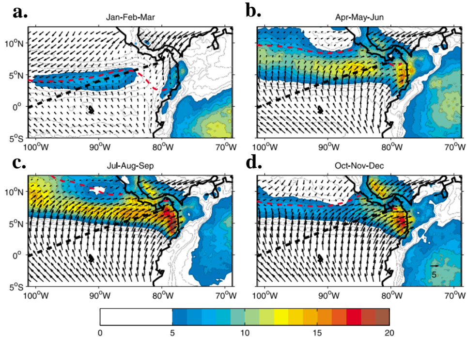
Figura 1. Climatología estacional (1999-2001) de vientos superficiales Quikscat (m/s, flechas) y precipitación TRMM (mm/día, colores). La ZCIT está definida donde los vientos convergen (línea roja discontinua). [Alory et al., 2012].
