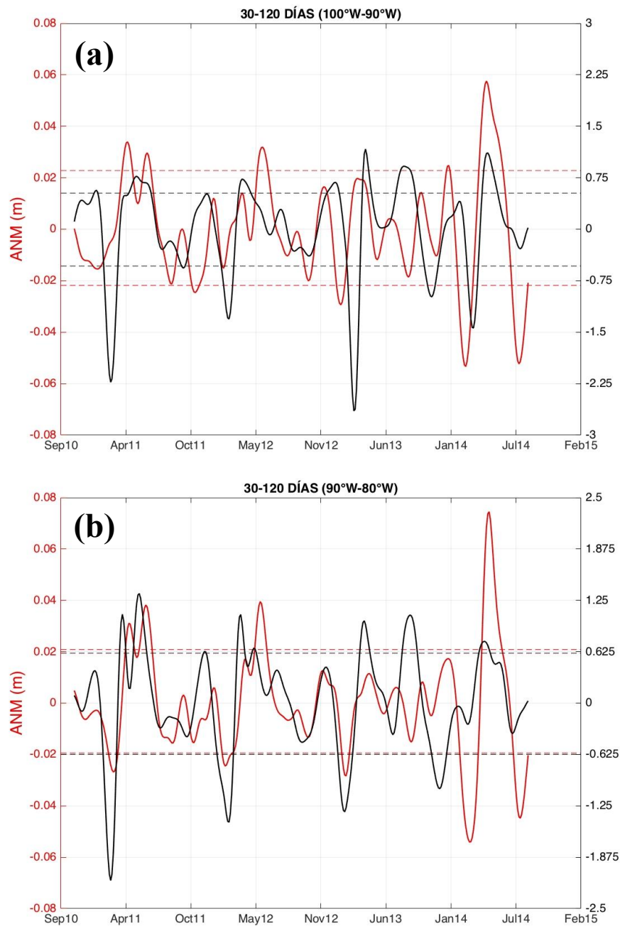
Figura 33. Serie de tiempo de la ANM (línea roja) y la posición del FE (línea negra) al (a) oeste y (b) al este de Galápagos luego de remover la señal de baja frecuencia ( > 120 días). Las líneas horizontales discontinuas rojas (negras) representan el límite de significancia del 95% superior e inferior para la ANM (FE).
